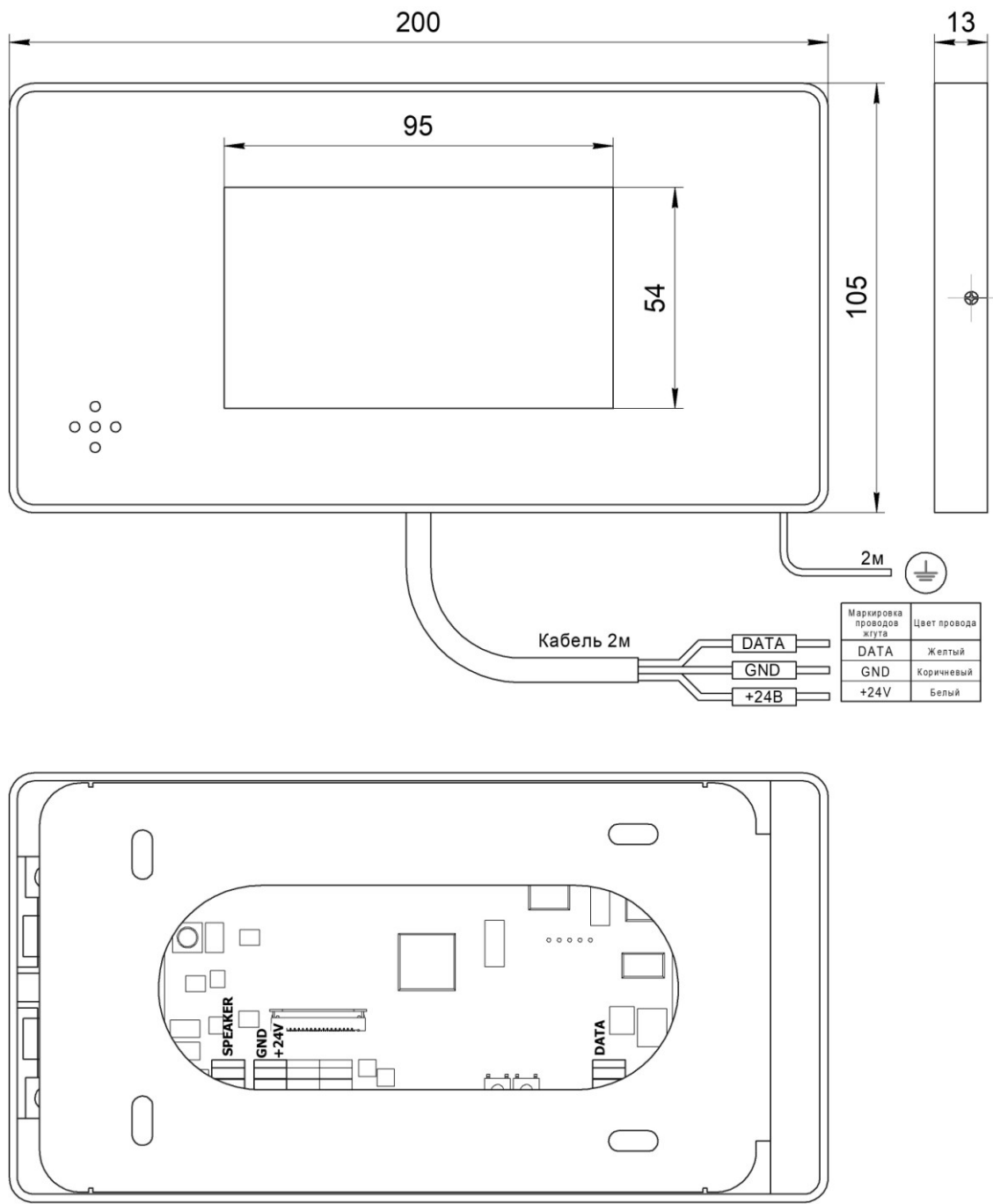
Рис.1 Внешний вид Табло накладное МАЛАХИТ НШЕК.468232.132-01 (дисплей 4,3 cPC)
